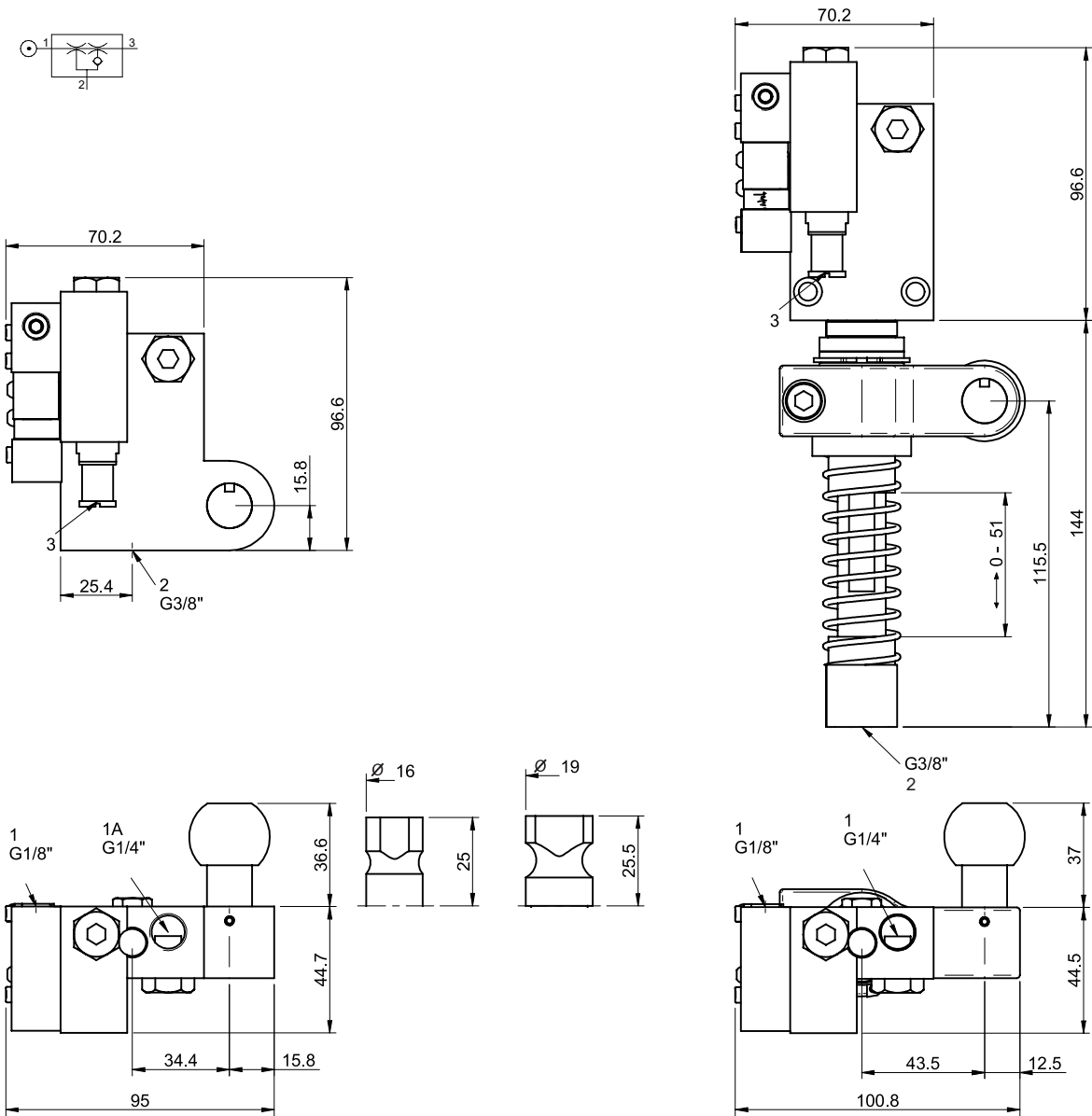
RYSUNEK WYMIAROWY
