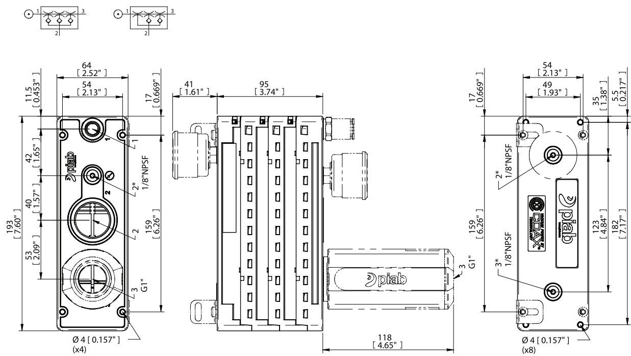
RYSUNEK WYMIAROWY
