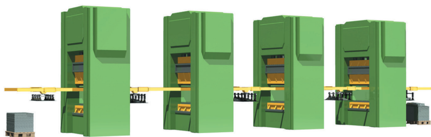
Podawanie arkuszy z prasy do prasy
