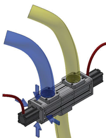
Przedmuch
