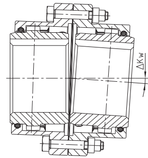
odchyłka kątowa
