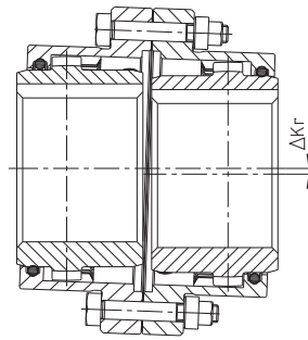
odchyłka promieniowa
