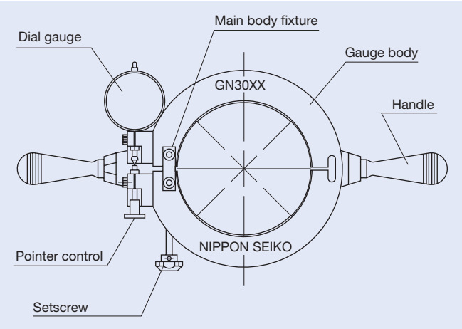
Fig. 1.9 GN Gauge
