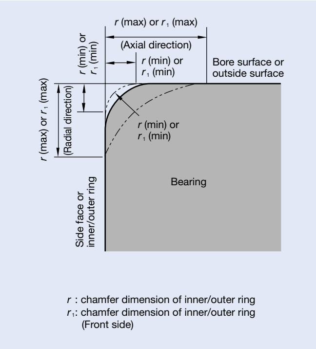
Fig. 8.2 Chamfer Dimension
